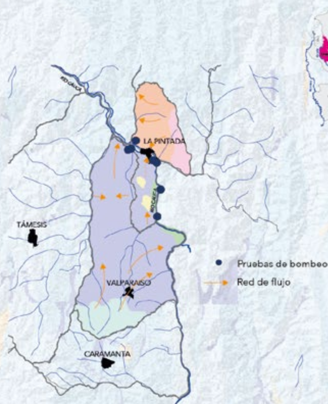
Zonas hidrogeológicas
