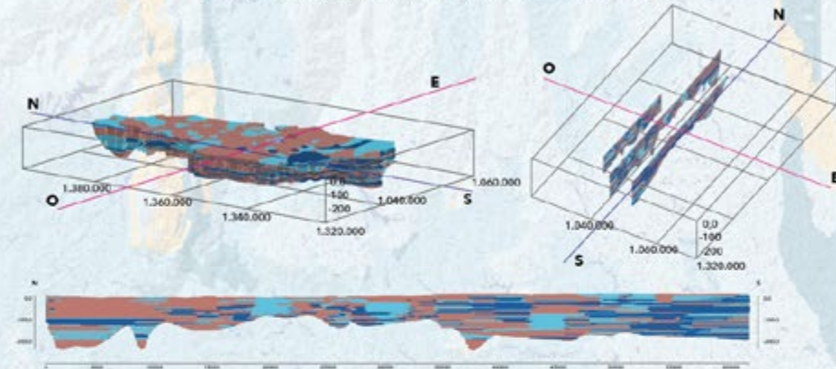
GEOMETRÍA DEL SISTEMA HIDROGEOLOGICO
