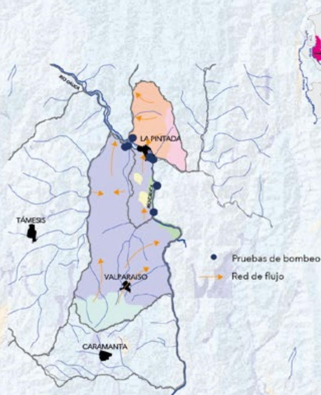
Zonas hidrogeológicas
