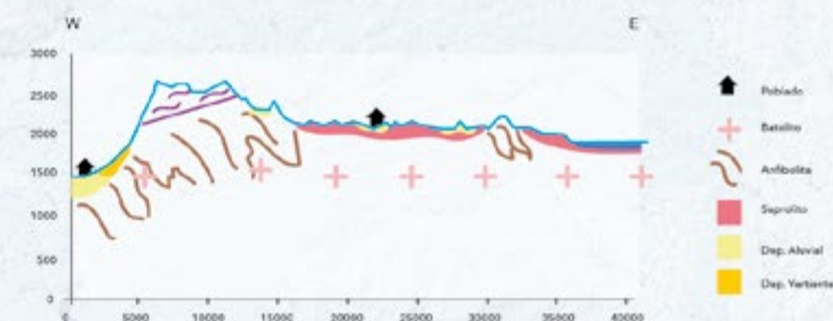
Perfil geológico de los Valles de Aburrá, San Nicolás y la superficie de erosión de El Peñol - Guatapé
