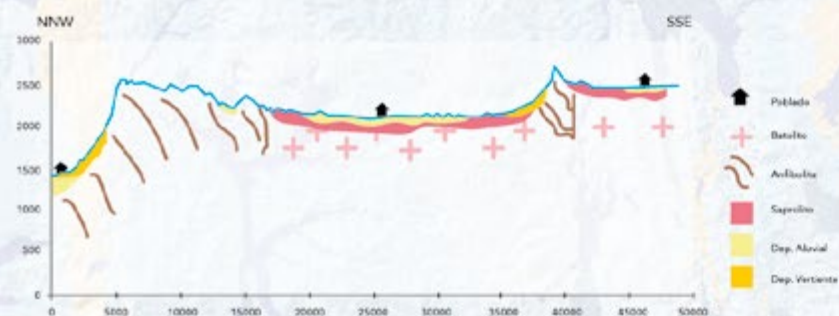
Perfil geológico de los Valles de Aburrá, San Nicolás y de La Unión en dirección NNW - SSE
