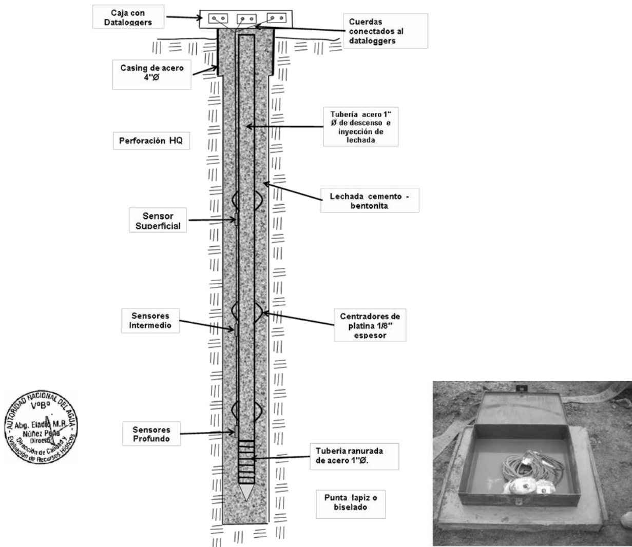
Figura 9 Piezómetro de Cuerda Vibrante
